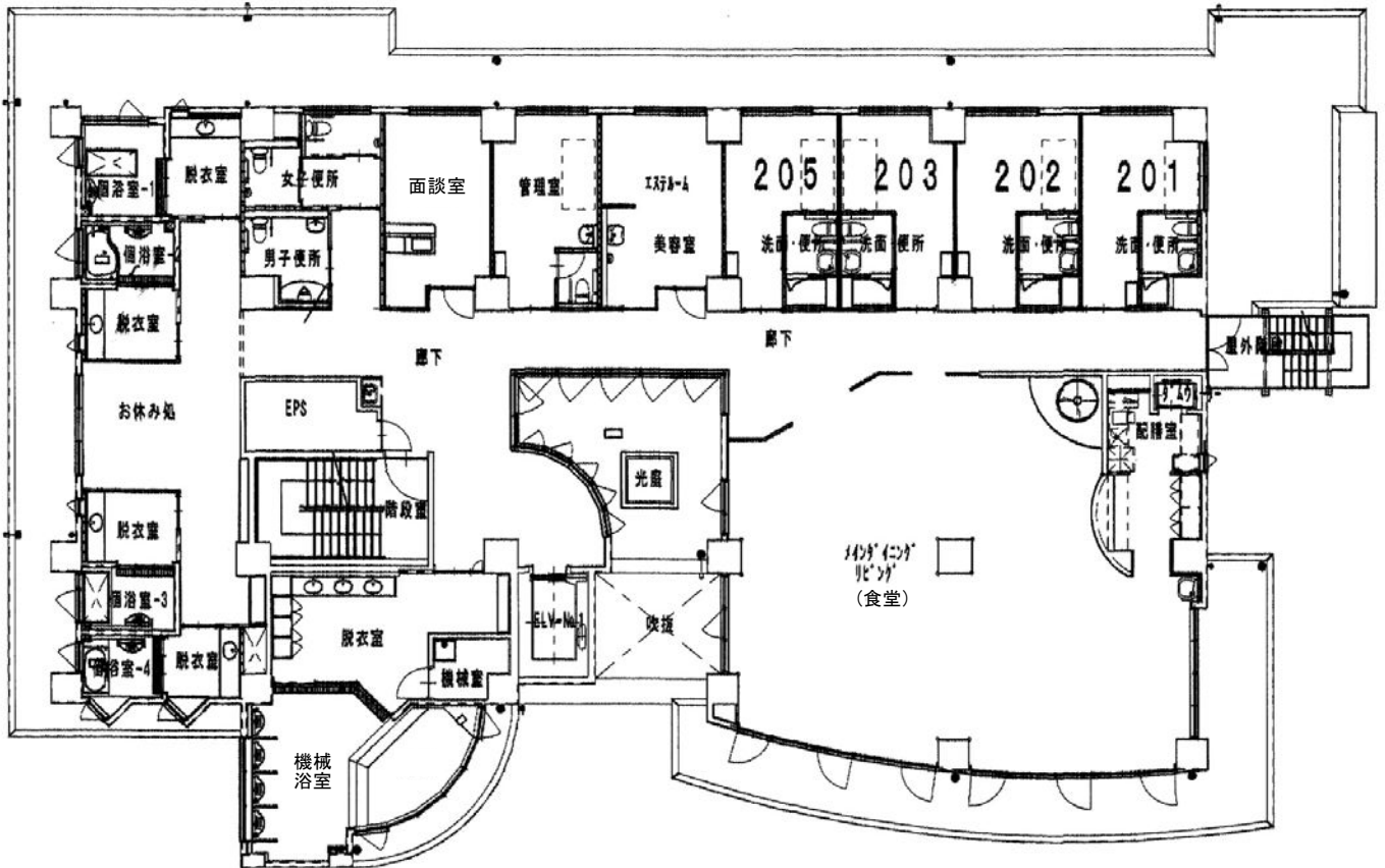
シニアあしたば 2階平面図
