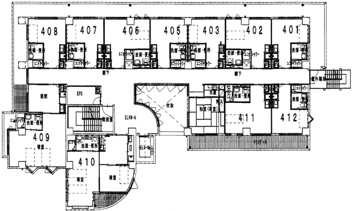
シニアあしたば 4階平面図
